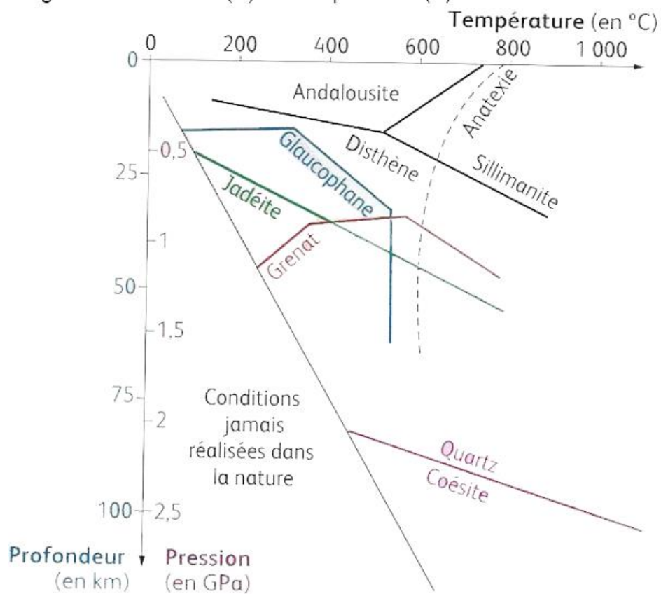
Diagramme Pression (P) et Température (T) des domaines de stabilité de minéraux
